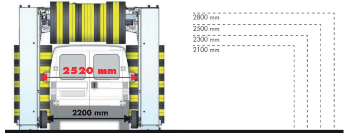
Largeurs de passage & hauteurs disponibles PORTIQUE S4
